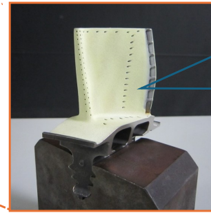
ガスタービン動翼
