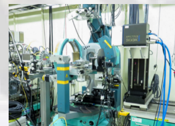
X線回折装置 (BL16XU) ※理研装置 薄膜材料、粉末材料、バルク材料などの構造解析、応力解析
