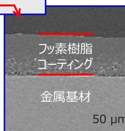
フッ素樹脂コーティング を施した自動車部品 www.sei-sfp.co.jp/products/fex.html
